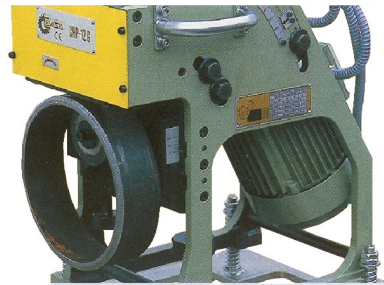
Pijpen afschuinen.
